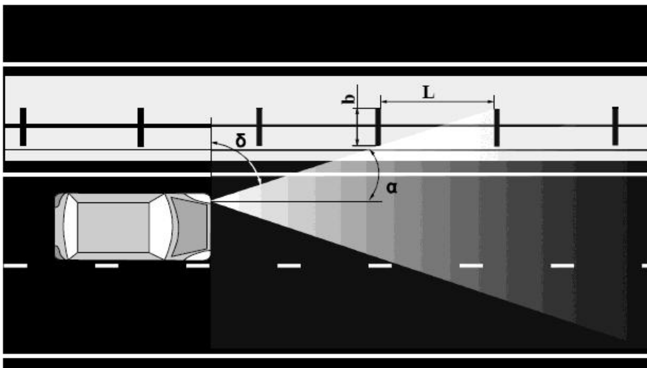
Рисунок 3 - Определение угла падения светового потока ( \alpha ) ограничивающего угла ( \delta ): b - ширина затемняющего элемента; L - расстояние между затемняющими элементами
